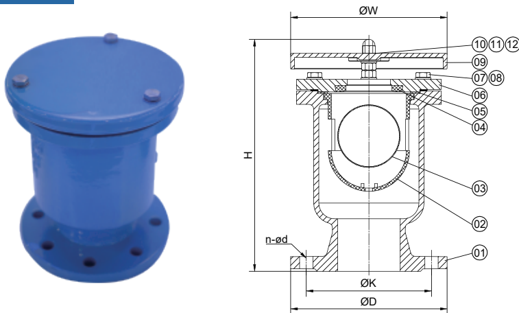
DN50-200
